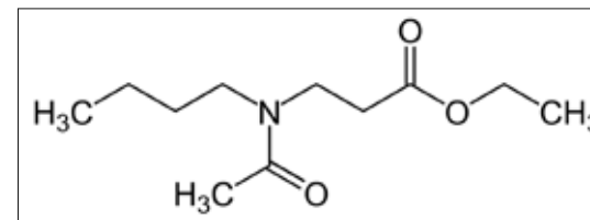
圖2 IR3535的 化學結構
