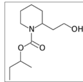
圖1 埃卡瑞丁的化學結構
